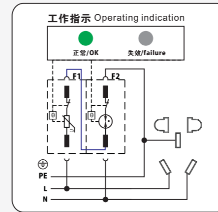
基本原理图 (Circuit Diagram) L-N,N-PE (1+1) mode
