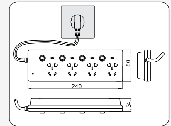
外形尺寸(Dimension):mm (WPX-SPA104)
